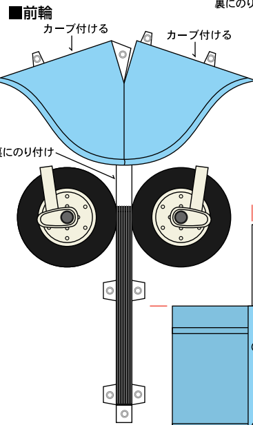
■前輪
